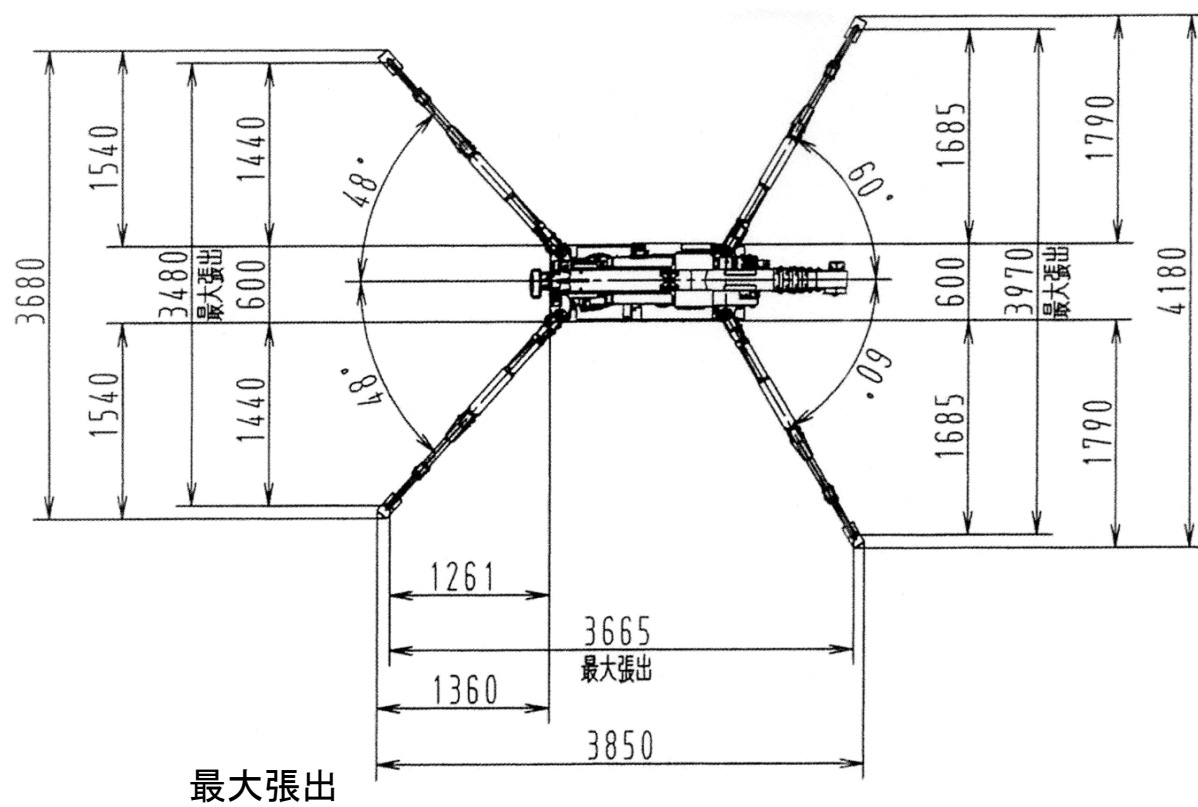
伏図
